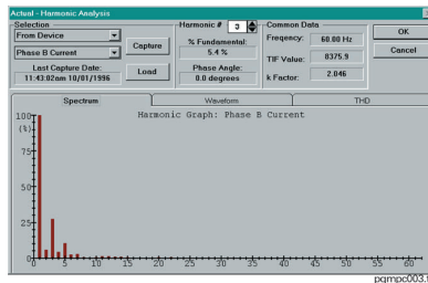
谐波波谱分析功能可以识别问题并确保正确地执行更改
