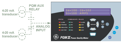
连接两个4~20mA变送器，用于过程变量测量和控制
