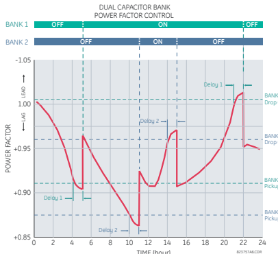
功率因数整定值和两个输出继电器可用于两级电容器组切换
