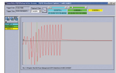
电压和电流波形可对系统问题分析提供有价值信息
