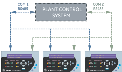
由第二个RS485通讯接口提供的高安全性系统中的冗余配置
